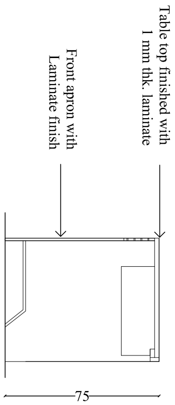
Elevation A
